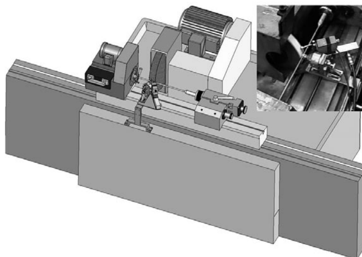
Фиг. 4 Надлъжно шлифване на нестабилен детайл с ръчно поднастроиваем люнет и използване на УАК
