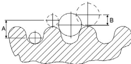
Фиг. 3 Различни отклонения на измервателните крайници при различен диаметър на контактните ролки
